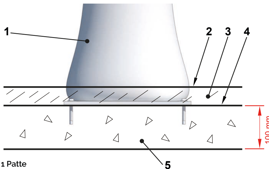
Détail d'ancrage
