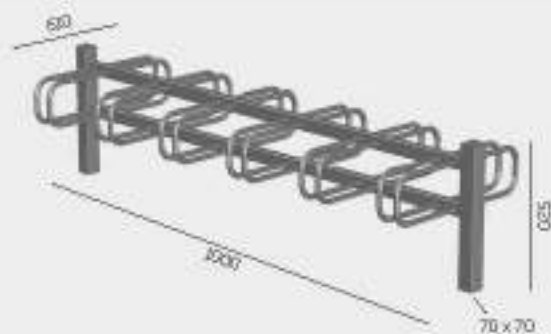
PV 381 TÊTE PLATE - 2 X 6 PLACES
