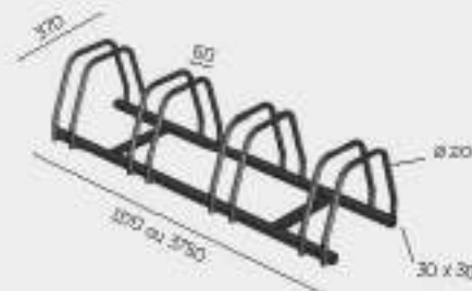
PV 20 APPUIS VELOS À CHEVILLER - 4 PLACES PV 20-1 : 11 PLACES
